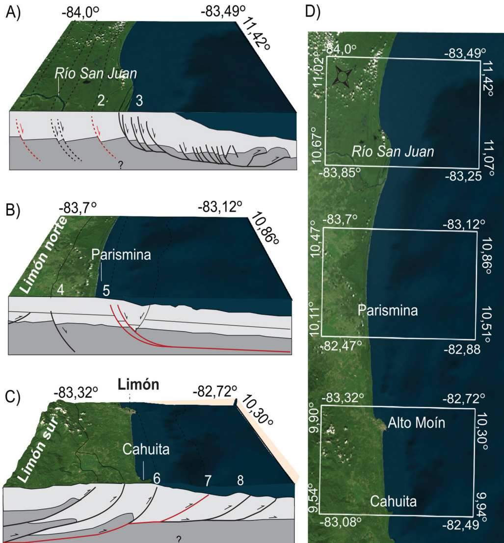
Fig. 2: Bloques esquemáticos que muestran las principales estructuras en el Caribe de Costa Rica, usados para definir planos de ruptura (p.ej. rumbo y buzamiento). A) Zona de San Juan. B) Zona de Parismina C) Zona de Cahuita. D) Los polígonos blancos muestran la extensión de los bloques del panel izquierdo. Modificado de Brandes et al. (2007a). Los números blancos hacen referencia a los planos de ruptura seleccionados en este trabajo.
